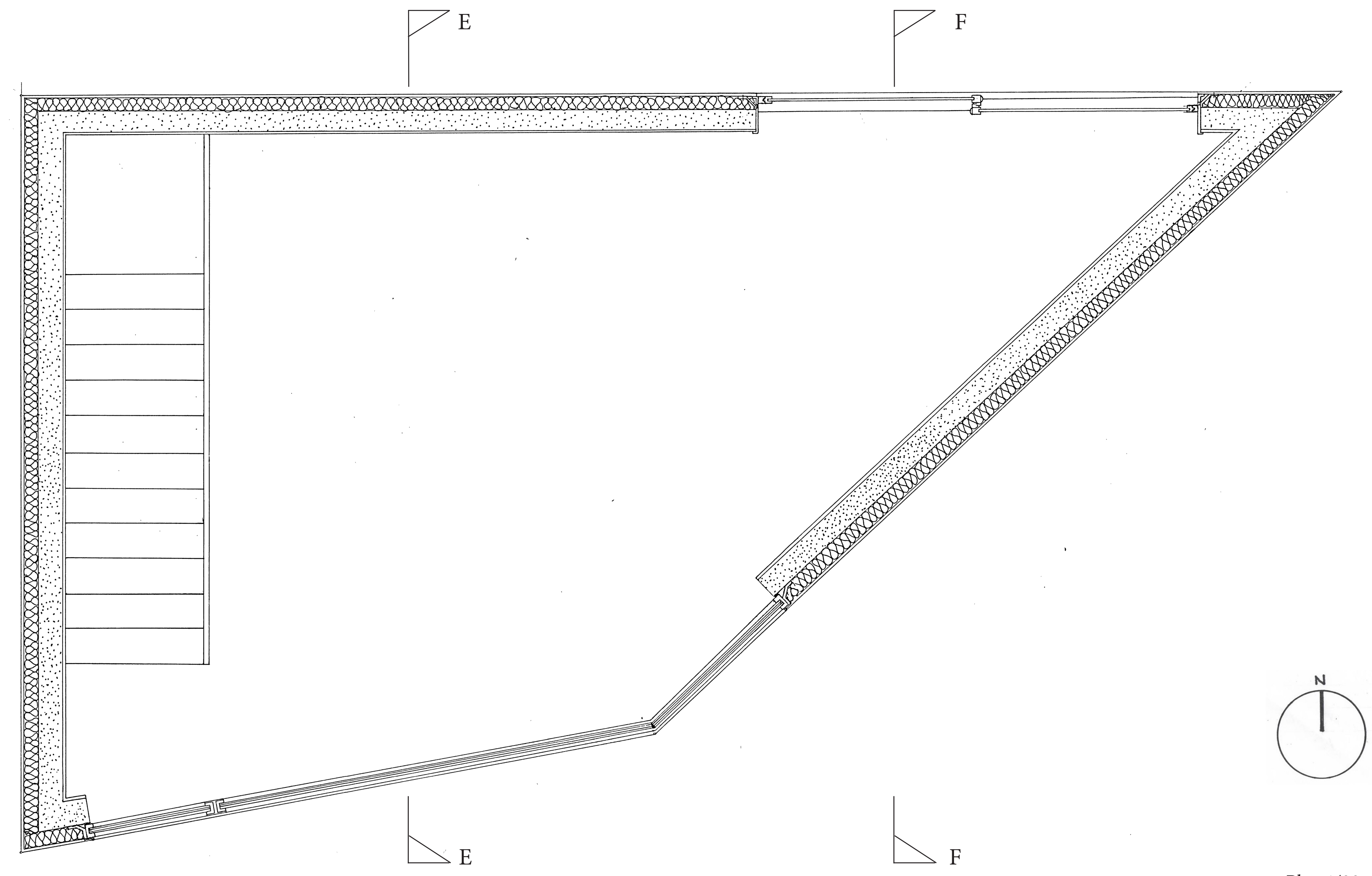
Plan 1/20
