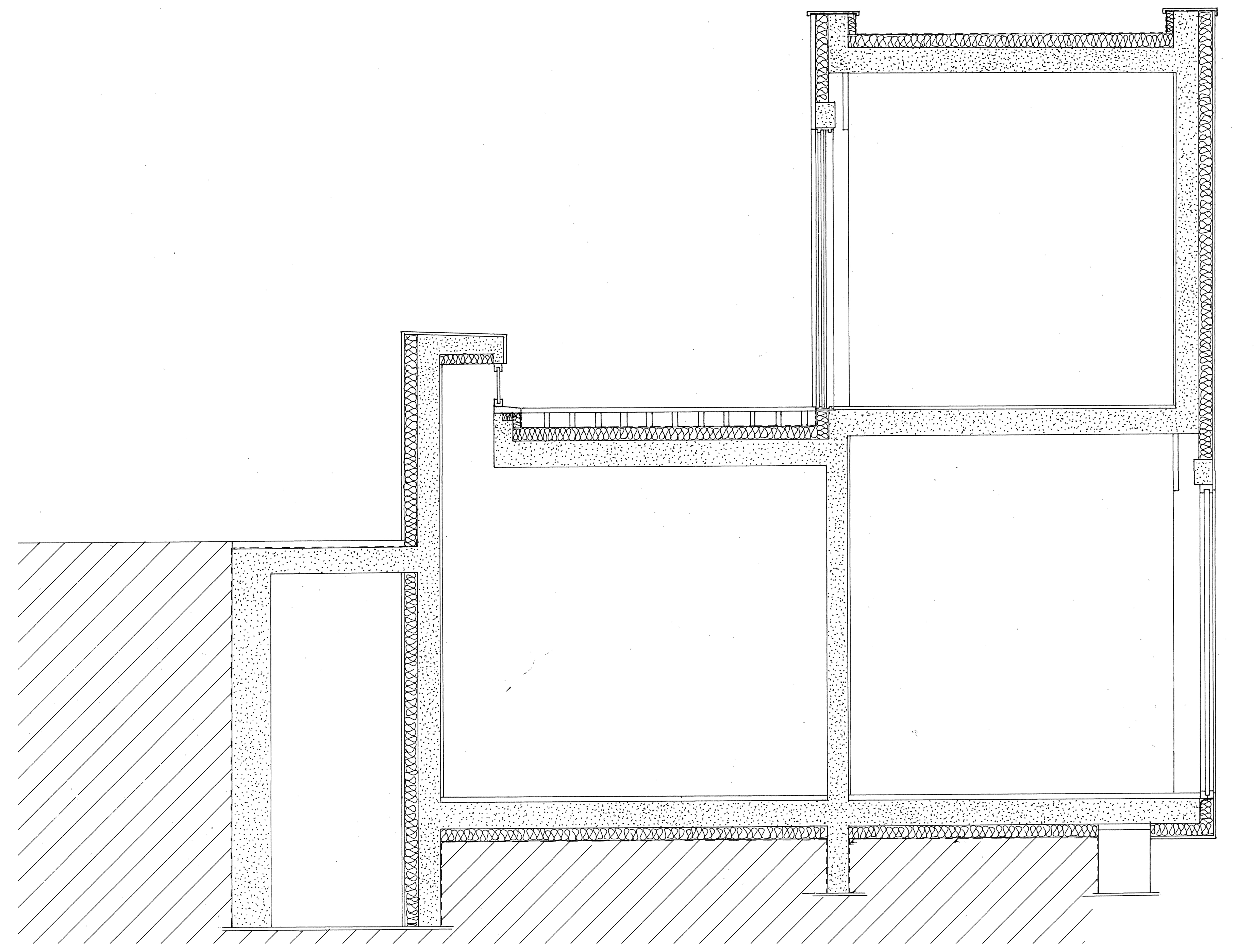
Coupe FF 1/20
