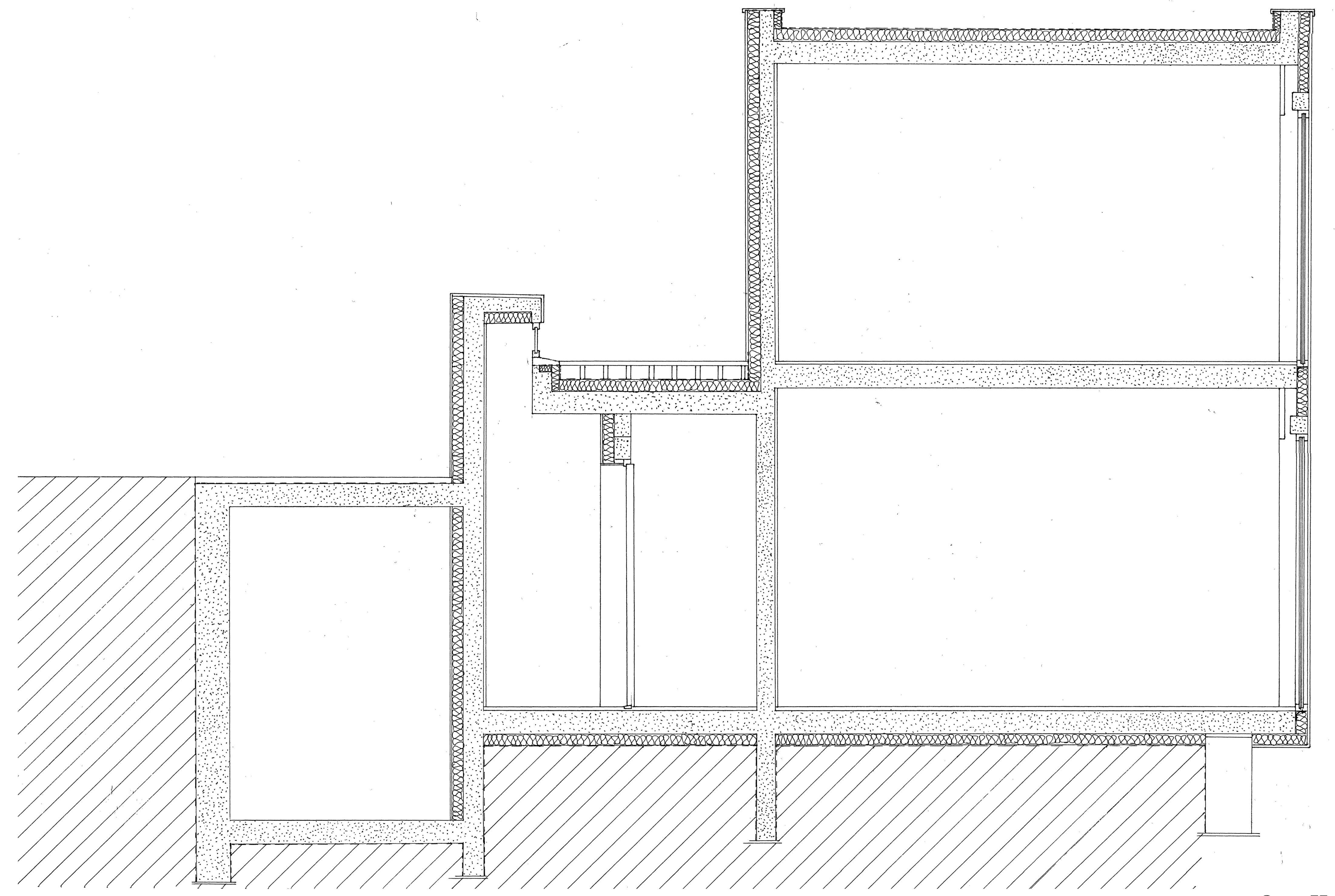
Coupe EE 1/20
