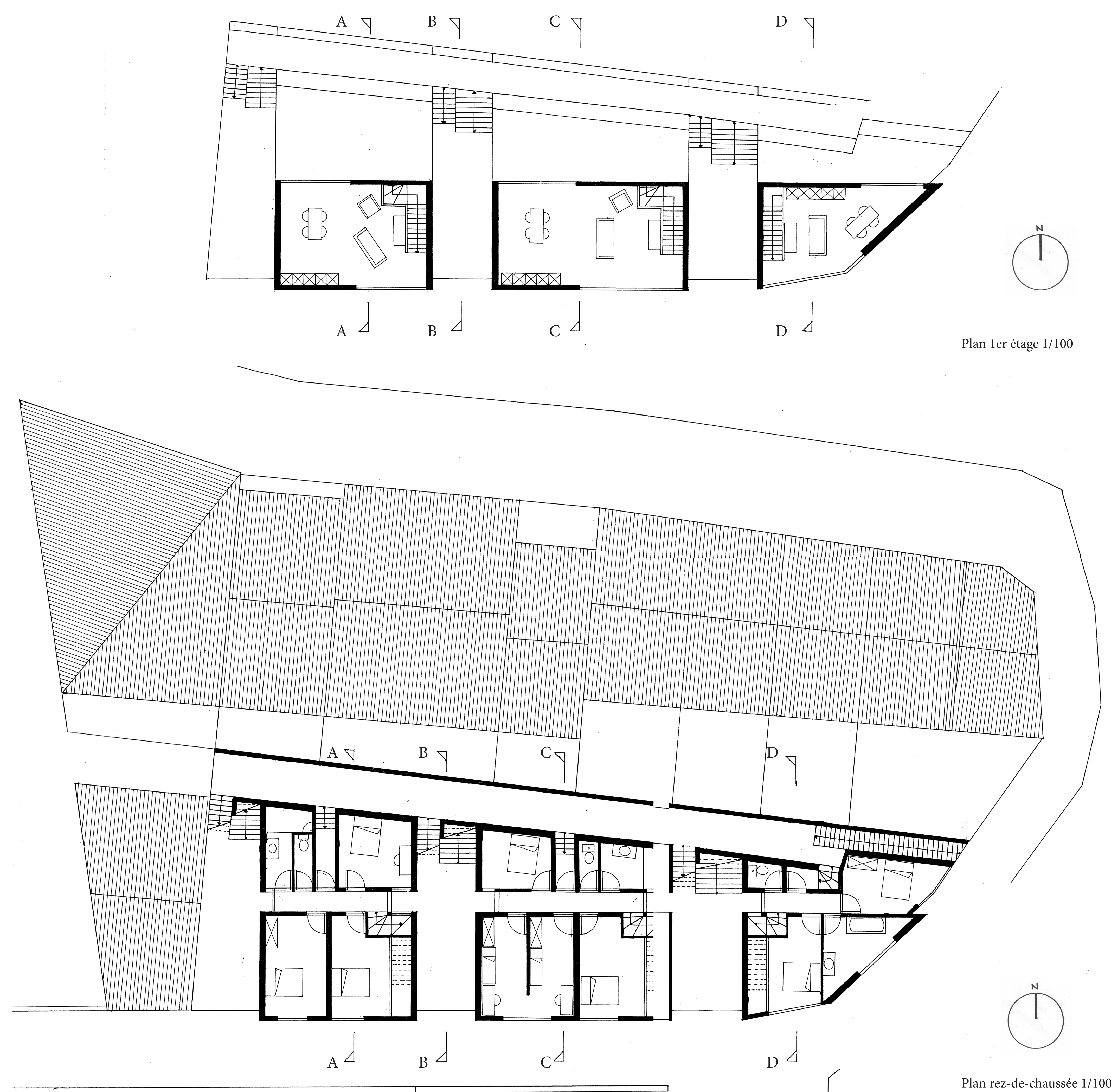
Plan 1er étage 1/100
