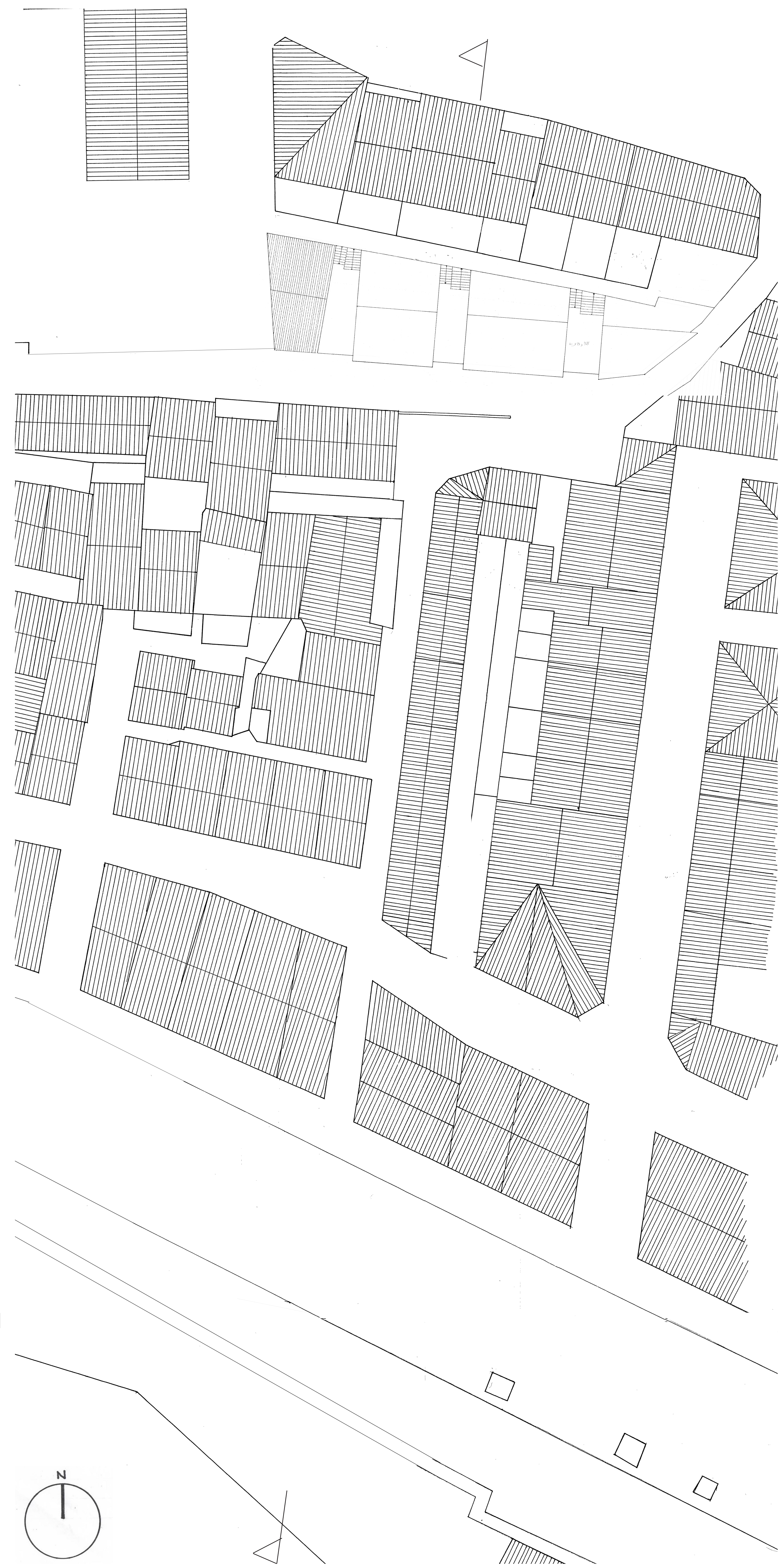
Plan masse 1/200
